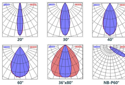
Diagramas fotométricos
